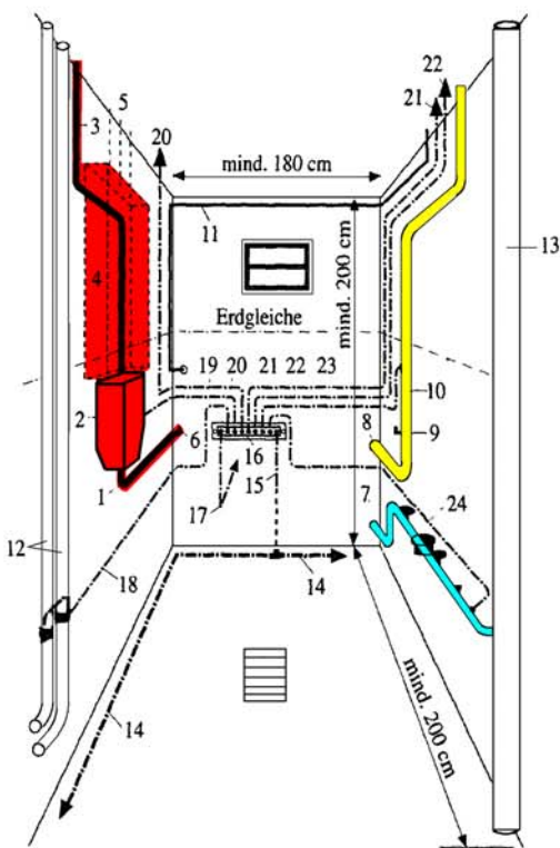
Bild 1: Hausanschlussraum nach DIN 18012
